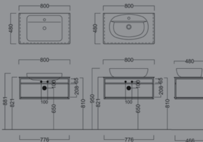
Метал. структура PLAZA Next, подвесная 80 см, цв. черный матовый PLAZA Next metal structure wall hung 80 cm, black matt
